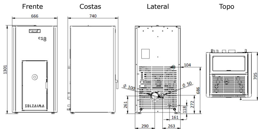
Figura 3 - Dimensões das caldeira Compacta Eco 18
