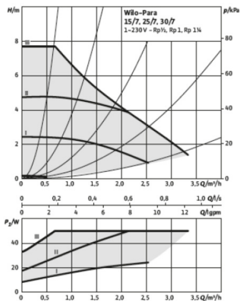
Figura 55 – Desempenho da bomba – Velocidades constantes I, II e III
