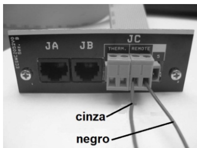
Figura 21 - Ligações do comando externo com fios
