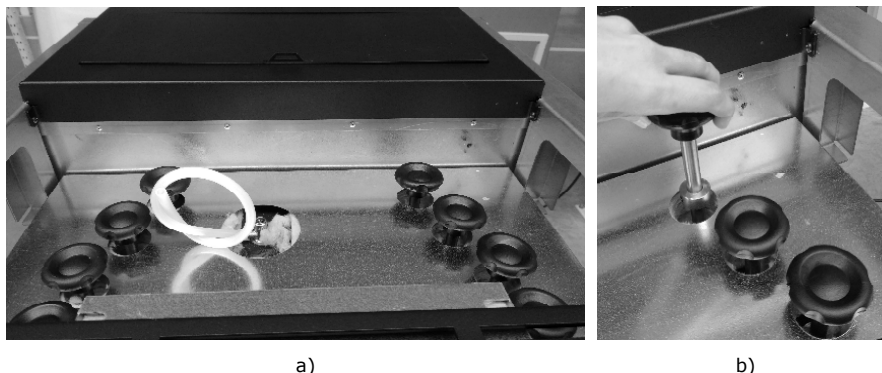
Figura 28 - Limpeza dos turbuladores
