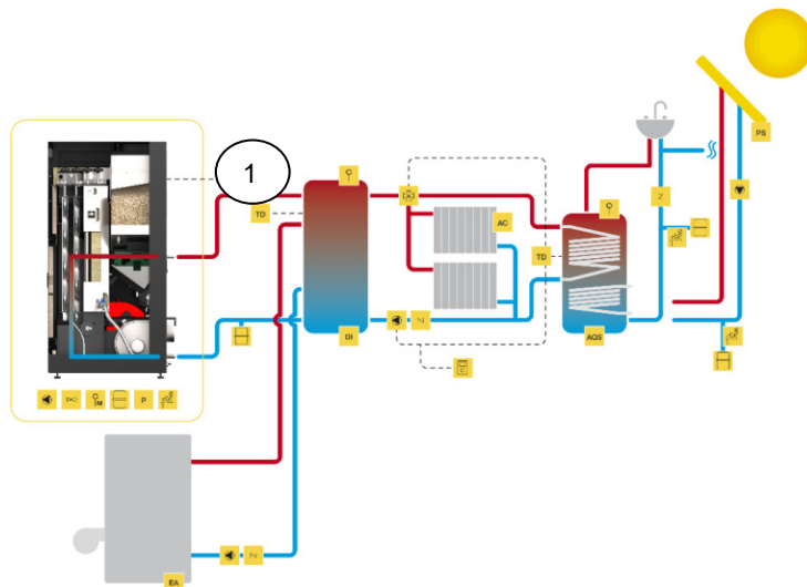
Figura 39 - Ligação a radiadores de aquecimento central, conjugado com outra caldeira de apoio e águas sanitárias combinado com painel solar
