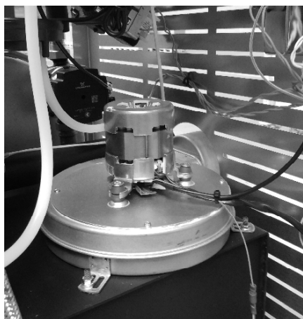
Figura 34 - a) Retirar os parafusos; b) Retirar extractor
