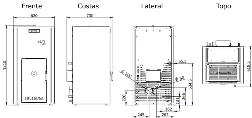
Figura 2 - Dimensões da caldeira Compacta Eco 12
