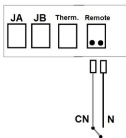
Figura 21 - Ligações do comando externo com fios
