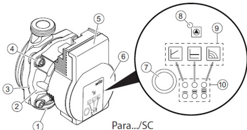
Figura 49 – Bomba Wilo
