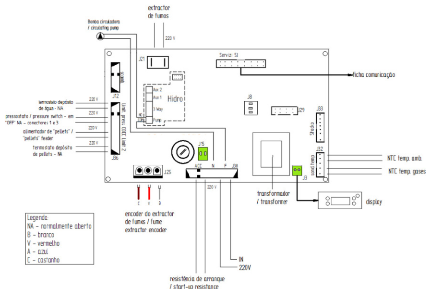
Figura 42 - Esquema eléctrico Compacta Eco 12
