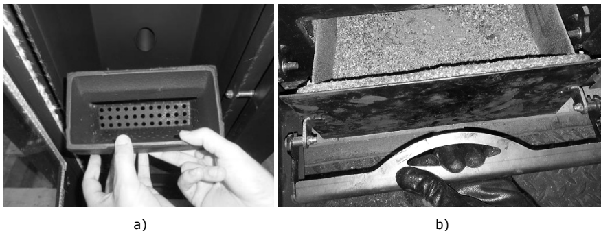
Figura 27 - a) Cesto de queima; b) Cesto de cinzas
