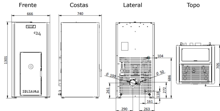
Figura 4 - Dimensões das caldeira Compacta Eco 24
