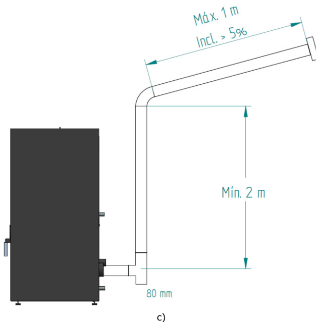
Figura 10 - Exemplos de instalações tipo
