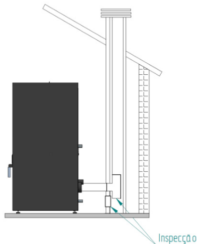
Figura 11 - Vista lateral da instalação com chaminé, com exemplo do ponto de inspeção
