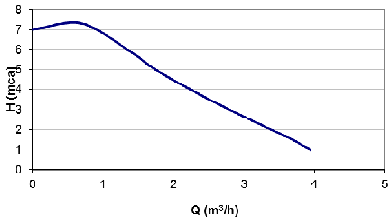
Figura 45 - Gráfico de desempenho da bomba
