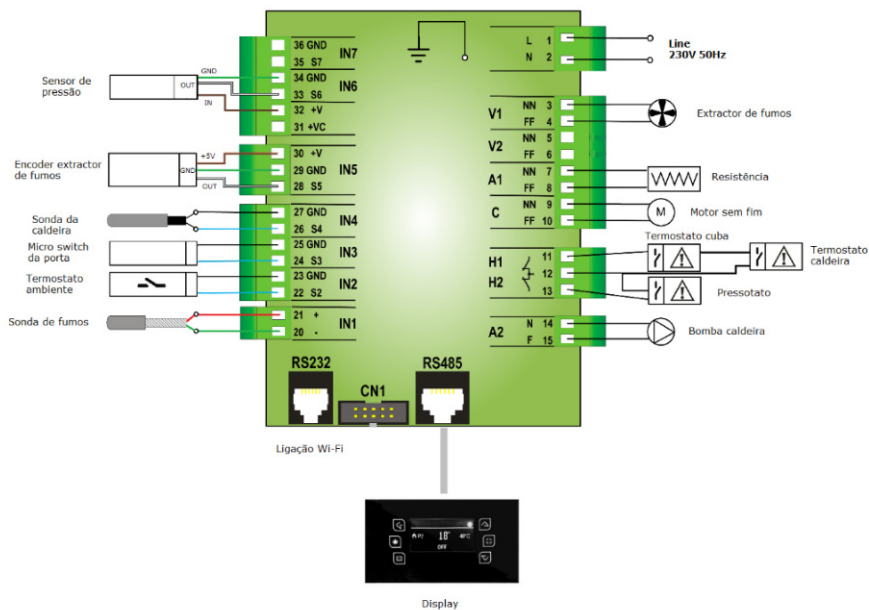
Figura 44 - Esquema eléctrico (eletrônica Columbus)
