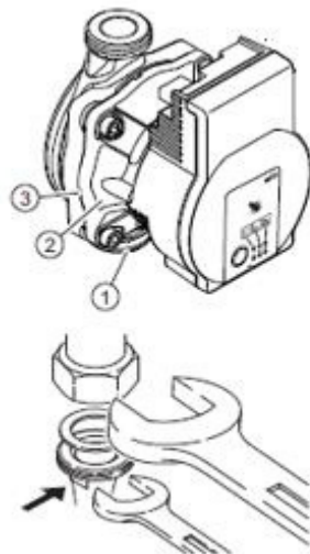
Figura 50 – Instalação da bomba
