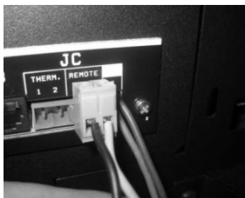
Figura 20 - Ligação do comando remoto sem fios
