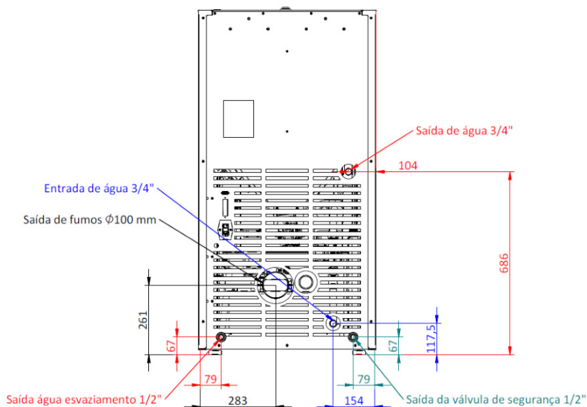
Figura 6 - Ligações hidráulicas das caldeira Compacta Eco 18 e 24
