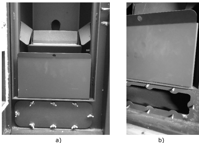
Figura 32 - Limpeza do interior da caldeira
