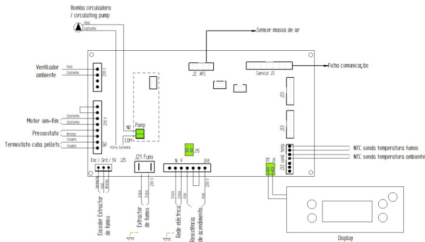
Figura 43 - Esquema eléctrico Compacta Eco 18 e 24
