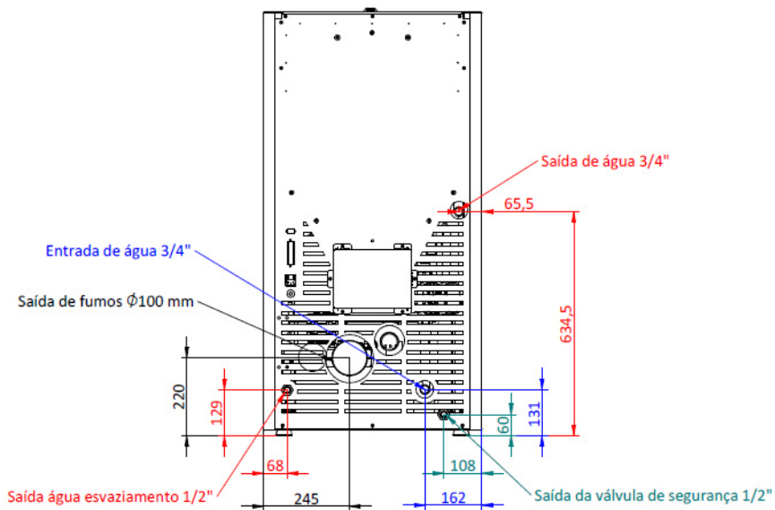
Figura 5 - Ligações hidráulicas da caldeira Compacta Eco 12
