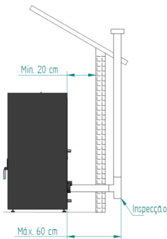
Figura 9 - Vista lateral da instalação sem chaminé, com exemplo do ponto de inspecção
