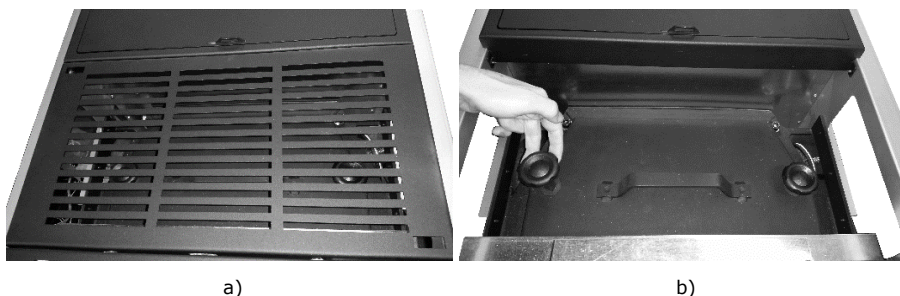
Figura 25 - Limpeza dos turbuladores
