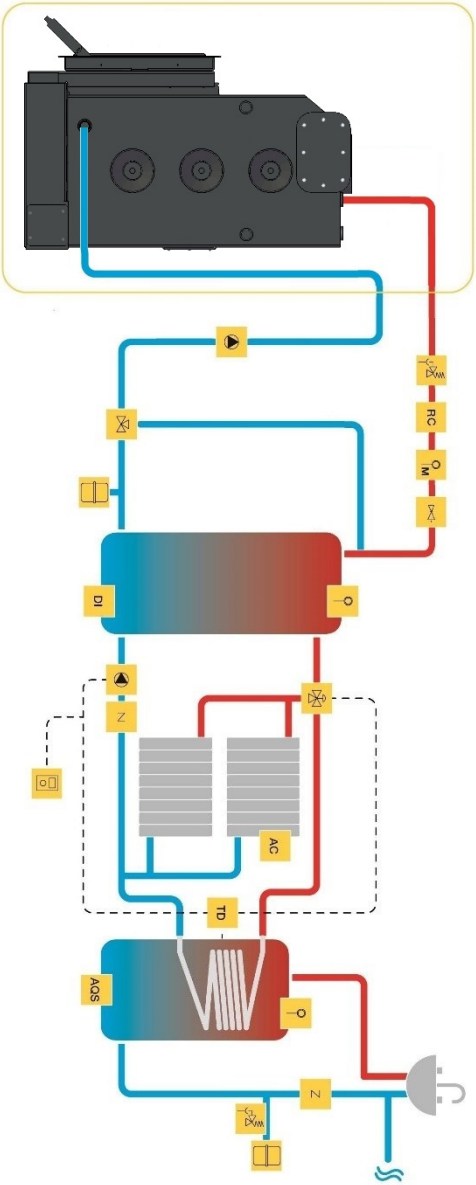
Esquema 2 – Instalação para aquecimento central (AC) e Águas Quentes Sanitárias (ACS)
