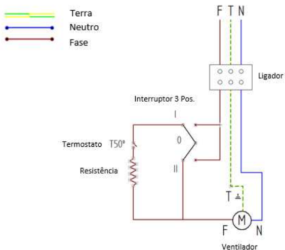
Figura 36 - Esquema Elétrico
