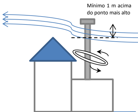
Figura 31 - Altura de chaminé correta
