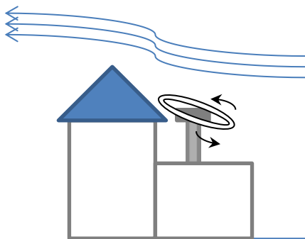
Figura 30 - Altura de chaminé incorreta
