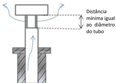
Figura 29 - União correta
