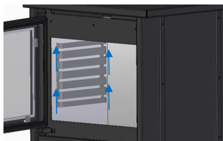
Figura 46 - Retirar grelhas laterais para limpeza do forno
