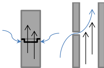
Figura 27 - Vedação incorreta
